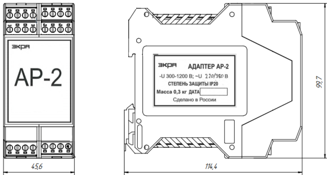
Рисунок 1 – Габаритные размеры адаптера реле AP-2
